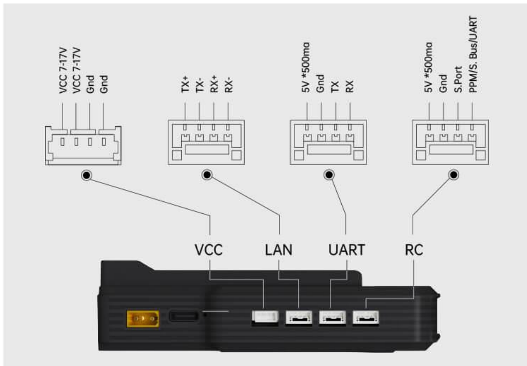
地面端接口定义
